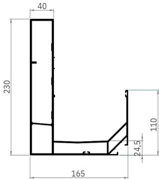
BEAM SECTION I SEZIONE TRAVE SECTION DE POUTRE I STÜTZBALKEN SECCIÓN DE LA VIGA I DRAAGBALKGEDEELTE
