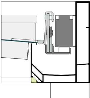
PERIMETER GUTTER I GRONDA PERIMETRALE GOUTTIÈRE PÉRIMÉTRIQUE I UMFANGSRINNE CANALÓN PERIMETRAL I DE GOTEN RONDON
